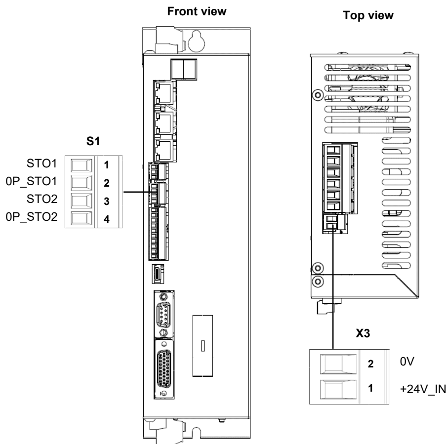
FIG. 2-Posizione dei morsetti X3 e S1 / Position of terminals board X3 and S1
